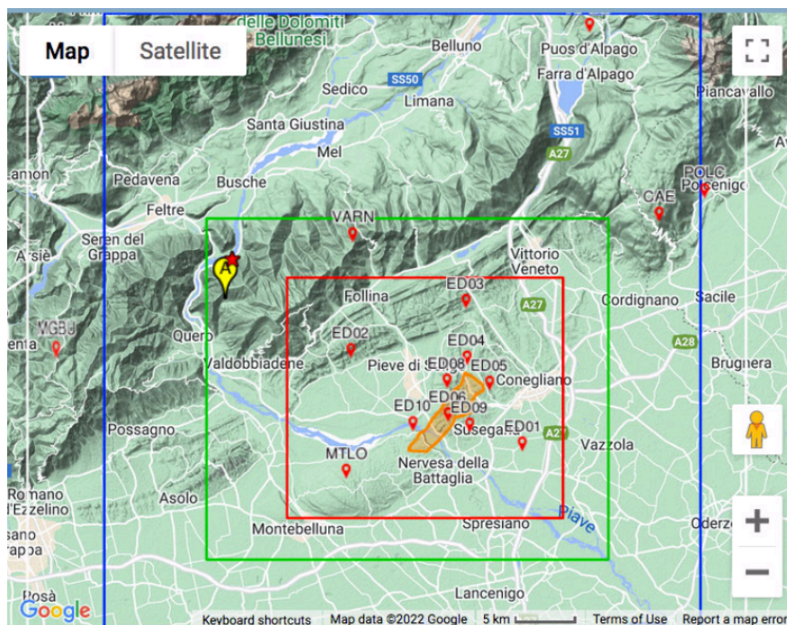
Figura 1 – Localizzazione dell’evento ML 2.3 del 5/8/2022 ora locale 07:37:39 (ora UTC 05:37:39). Nella figura sono rappresentate anche le stazioni sismiche utilizzate dal sistema di monitoraggio della RSC.
