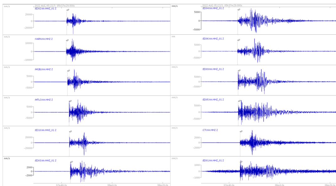
Figura 2 – Sismogrammi dell’evento ML 2.3 del 5/8/2022 ora locale 07:37:39 (ora UTC 05:37:39) registrati dalle stazioni utilizzate dal sistema di monitoraggio della RSC.
